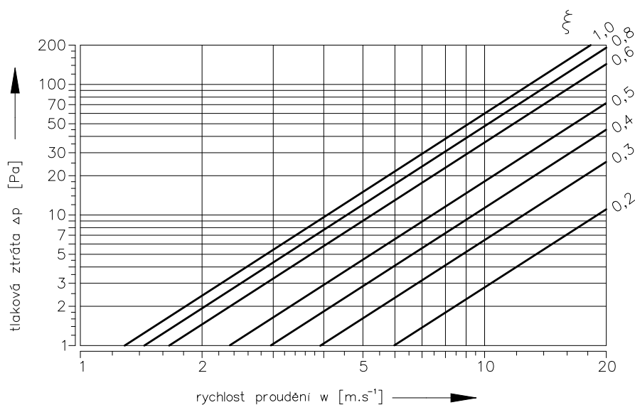
Diagram 5.2.1. Tlaková ztráta pro hustotu vzduchu
