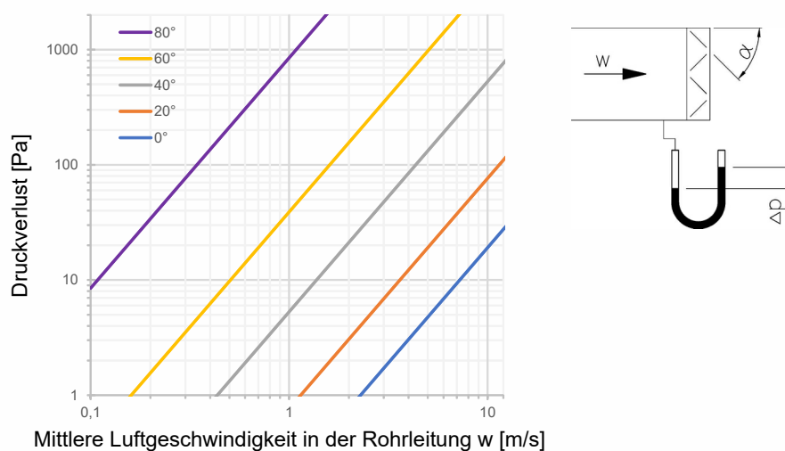
Diagramm 2 Regeldruckverlust in der Abhängigkeit vom Drehwinkel für Klappen, die Klappe in der Rohrleitung
