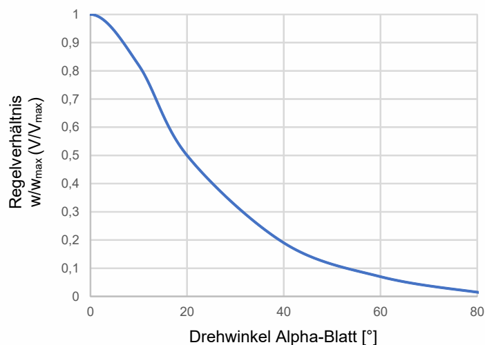
Diagramm 1 Durchflusskennlinie bei der ständigen Regeldruckdifferenz von 40 Pa
