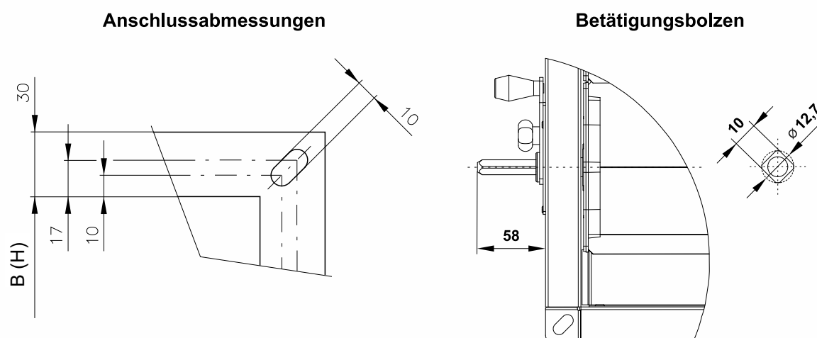
Abb. 6 Anschlussabmessungen
