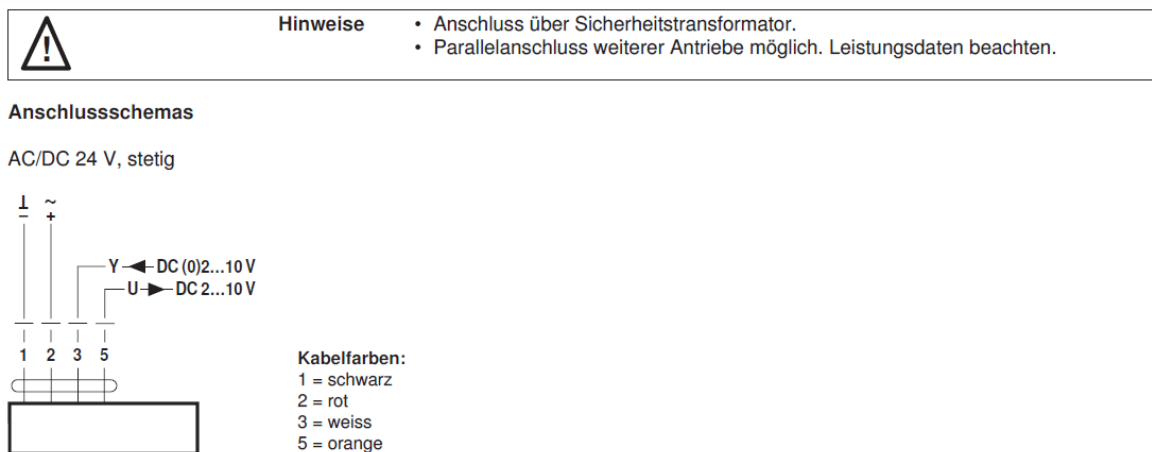
Abb. 9 Anschlussschema der Servoantriebe Belimo LM 24A-SR, NM 24A-SR, SM 24A-SR und GM 24SR.12
