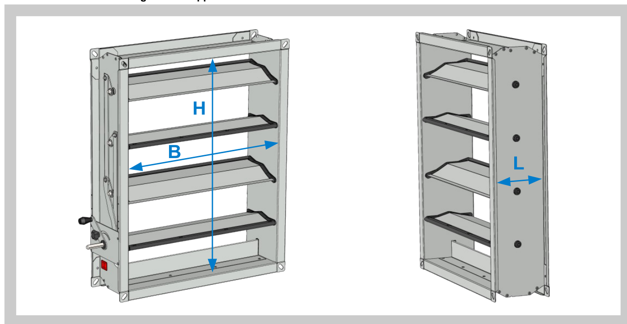
Abb. 1 Grundabmessungen der Klappe
