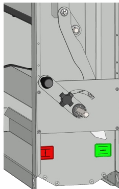
Abb. 3 Ausführung mit der Handbedienung und der Verriegelung
