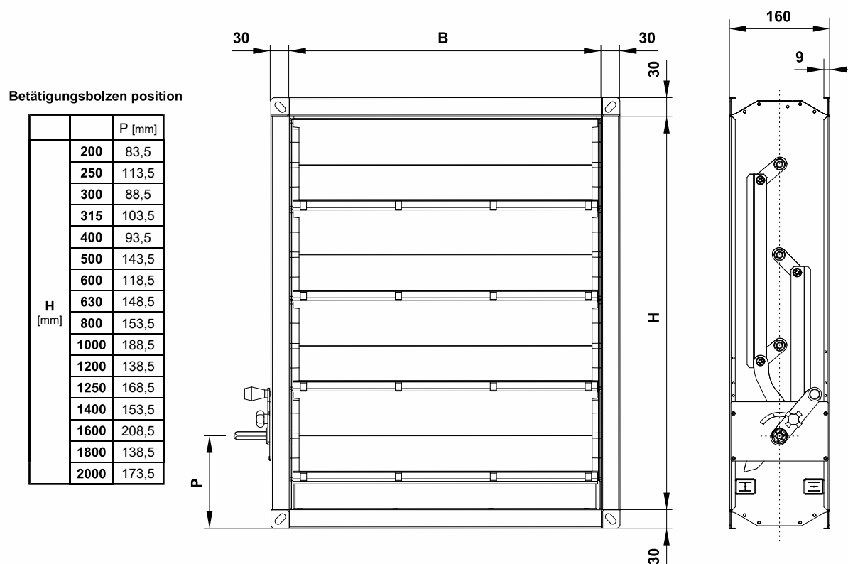
Abb. 5 Abmessungen der Klappe
