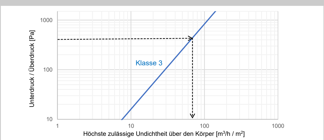
Diagramm 5 Dichtheit über geschlossene Blätter Klasse 3 nach EN 1751
