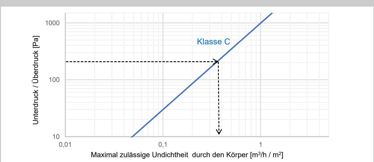
Diagramm 4 Dichtheit über den Körper Klasse C nach EN 1751
