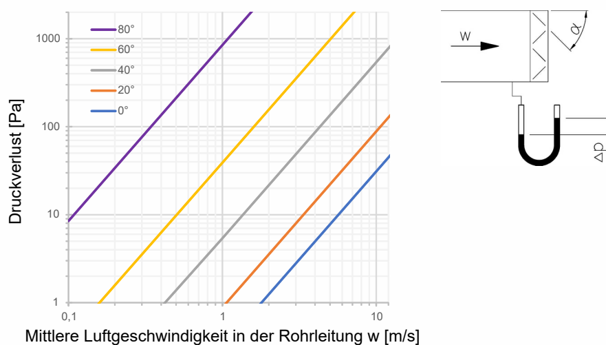
Diagramm 3 Regeldruckverlust in der Abhängigkeit vom Drehwinkel für Klappen, die Klappe am Ende der Rohrleitung
