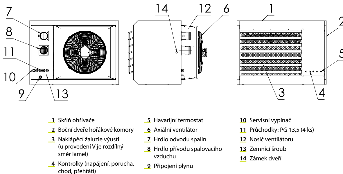
Obr. 4: Hlavní části ohřívače MONZUN Z(V)
