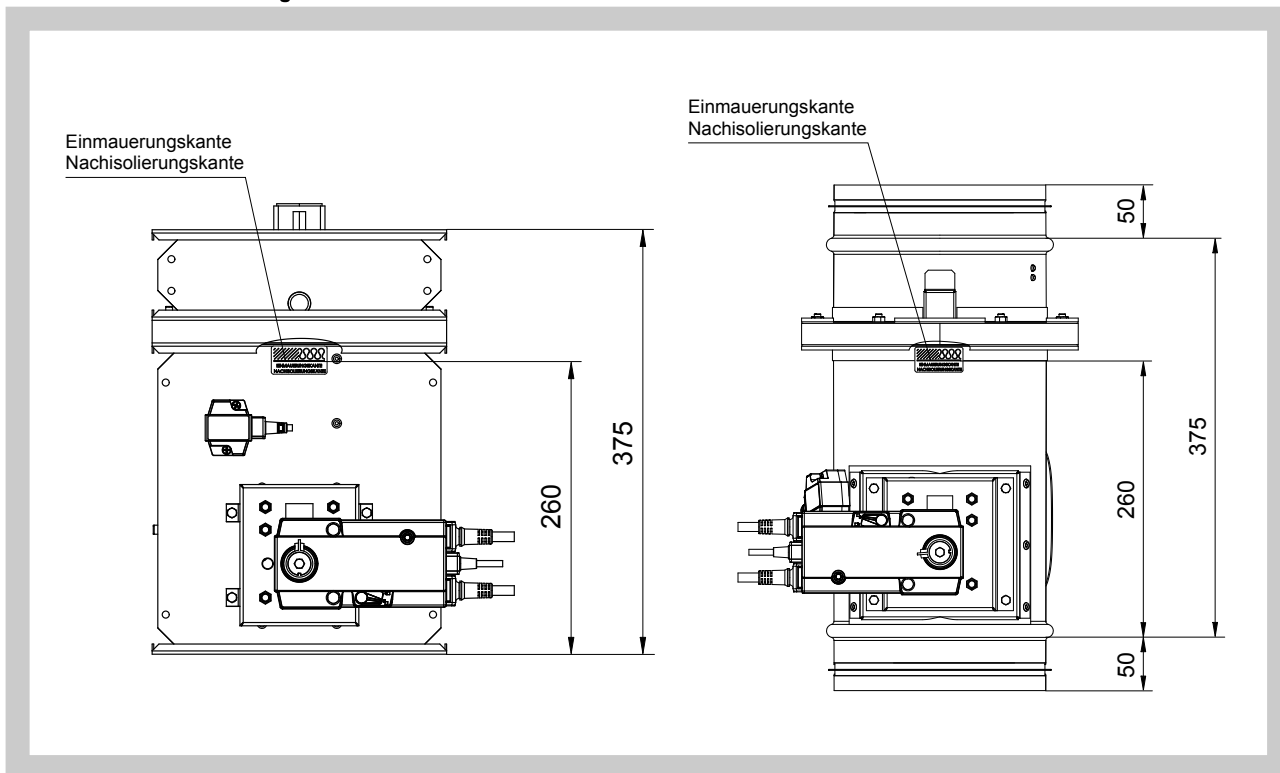
Abb. 43 Einmauerungskante
