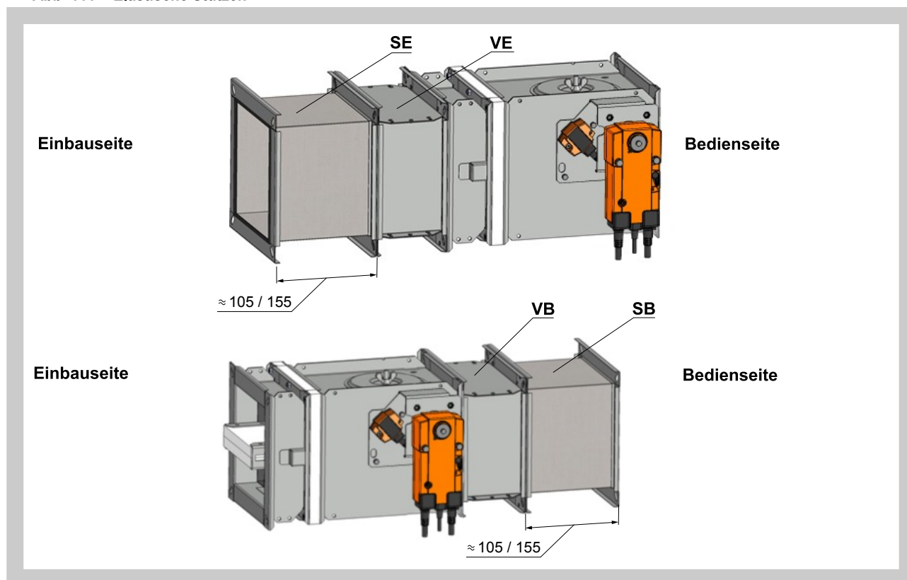
Abb. 111 Elastische Stutzen
