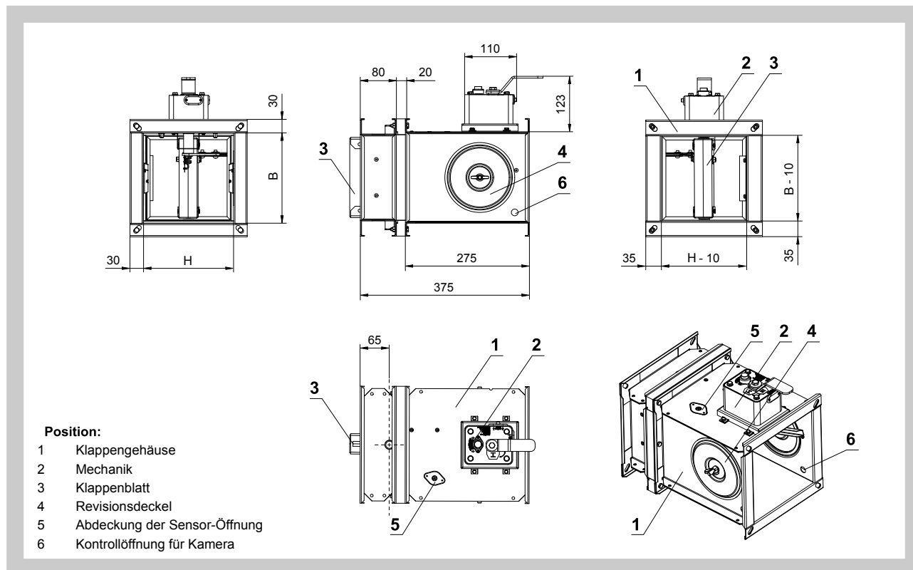
Abb. 30 MECHANISCHE AUSFÜHRUNG mit Schmelzlot
