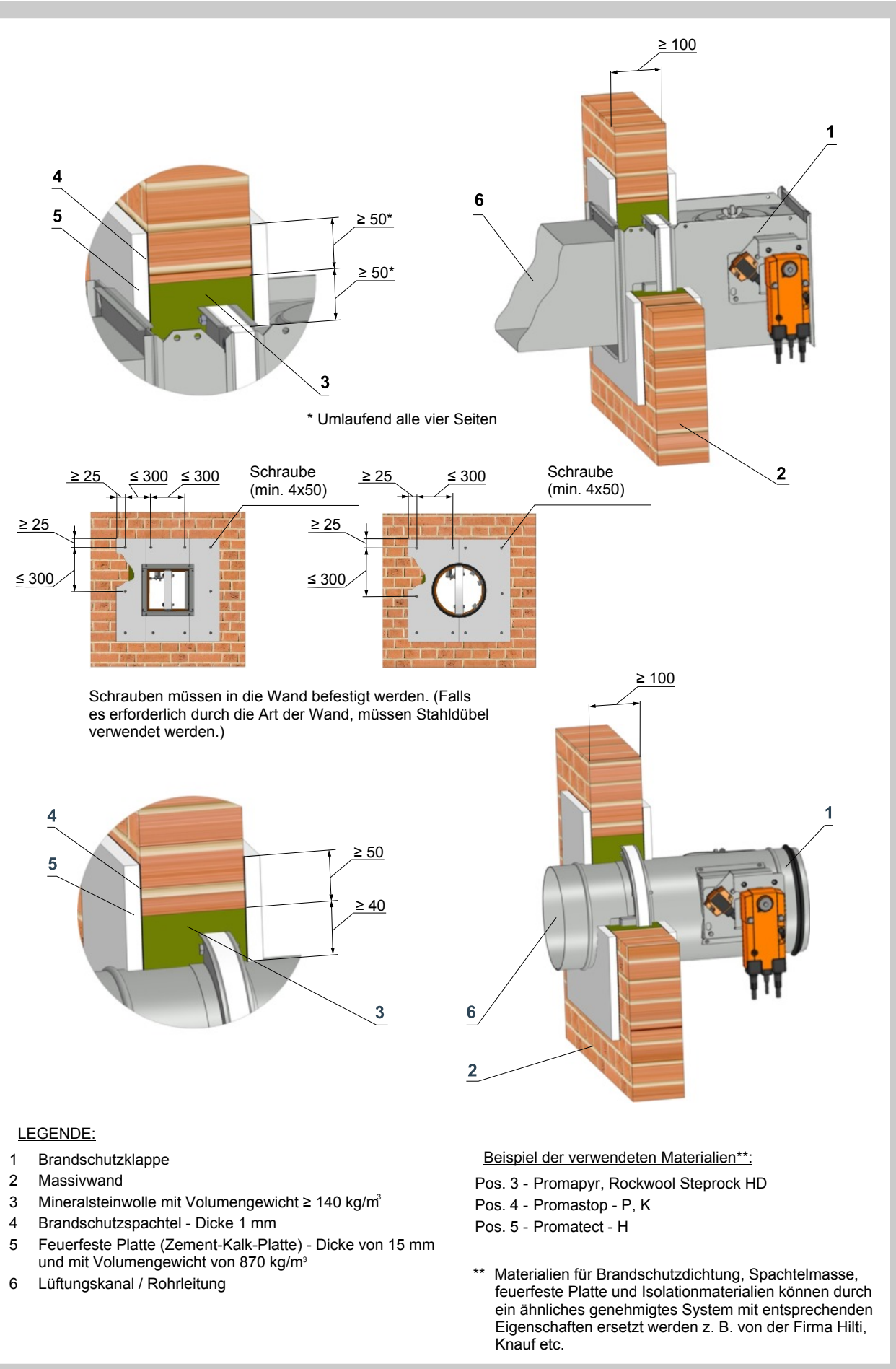
Abb. 54 Massivwände - Trockeneinbau - Brandschutzdichtung mit Spachtelmasse und feuerfeste Platte
