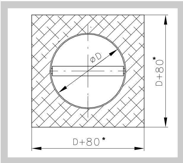
Abb. 46 Runde Klappen
