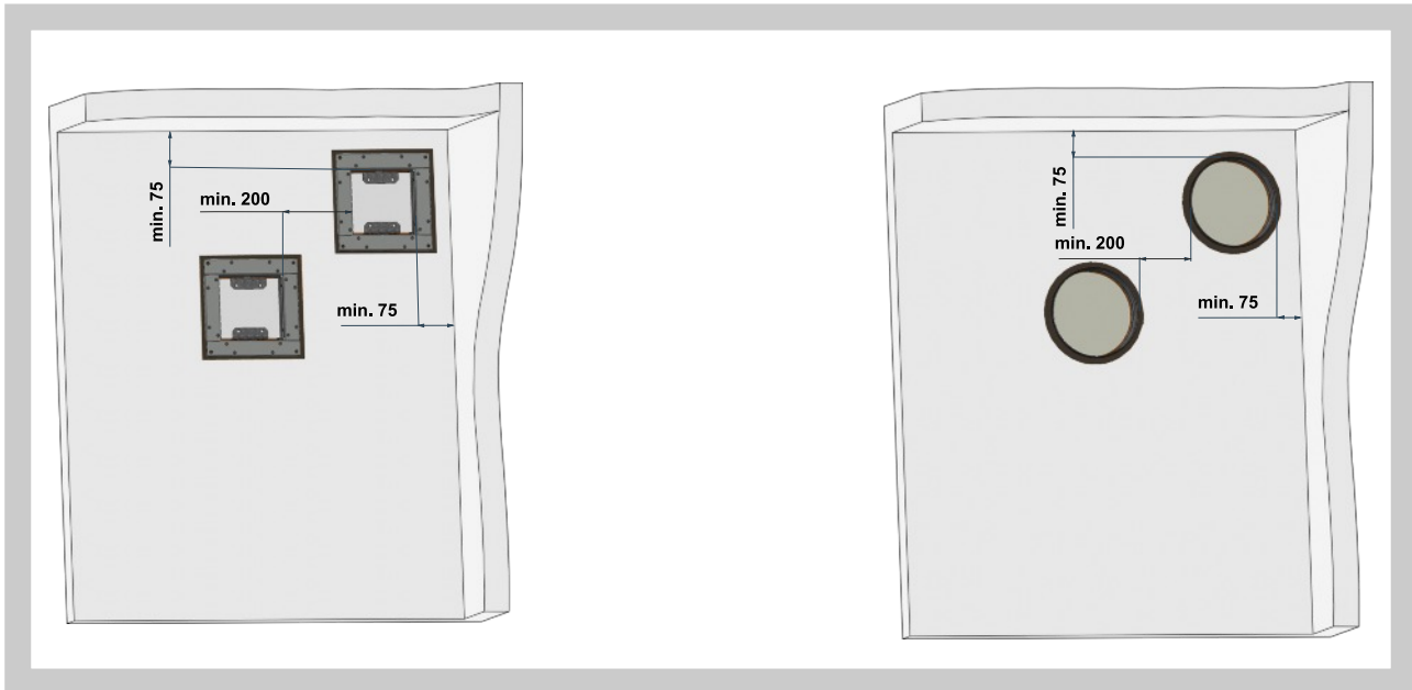
Abb. 42 Abstand zwischen den Brandschutzklappen und der Tragkonstruktion
