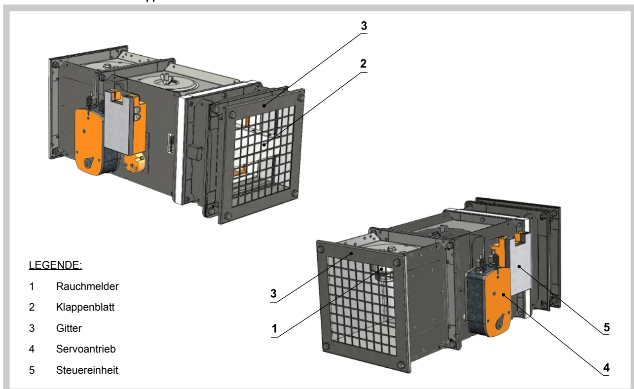
Abb. 116 Überströmklappe
