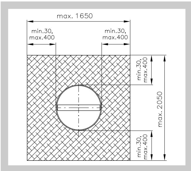
Abb. 48 Runde Klappen-Weichschott
