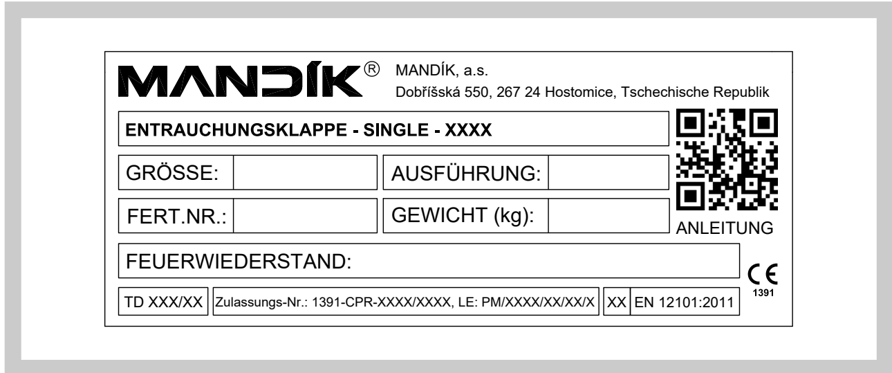
Abb. 9 Typenschild
