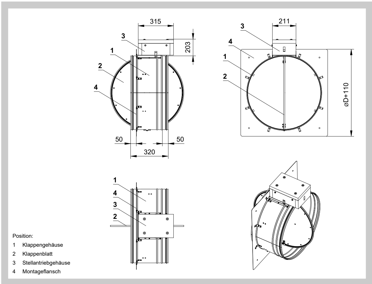
Abb. 6 Klappe SEDS-R
