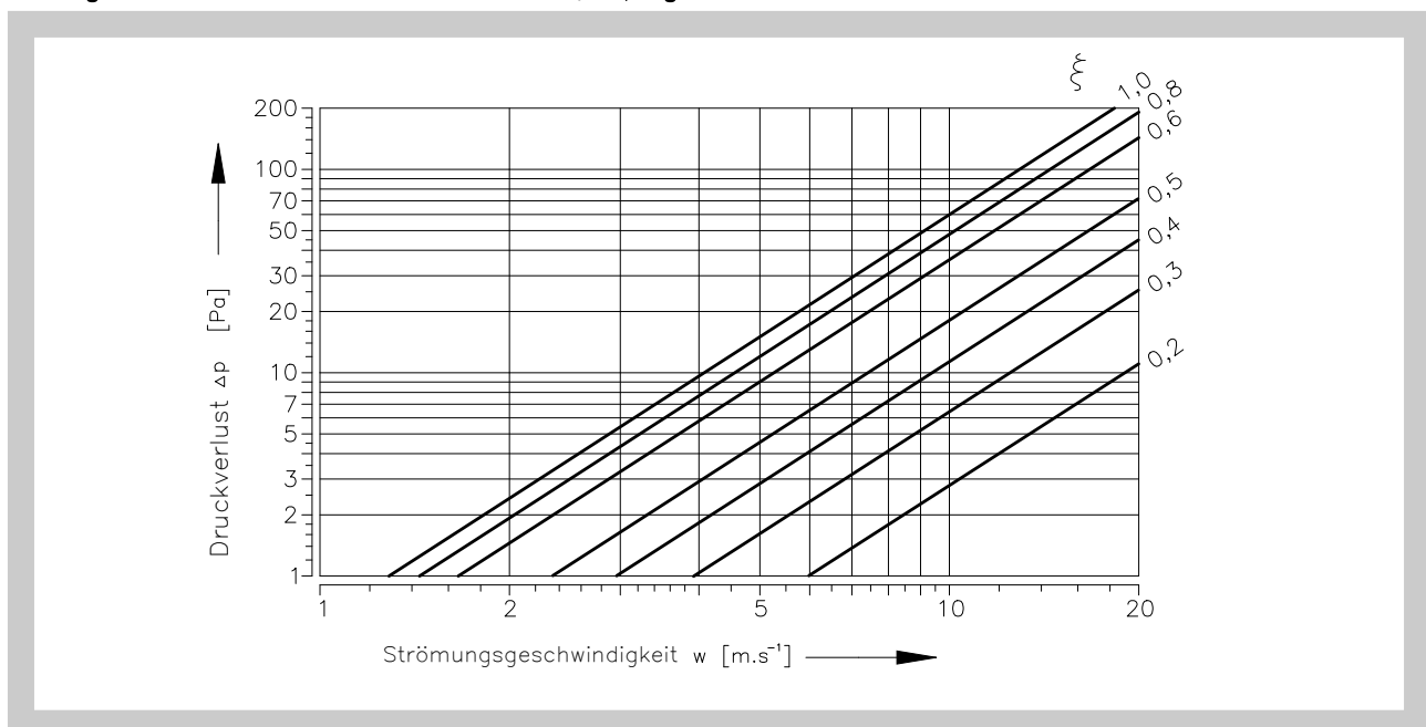
Diagram 1 Druckverlust für die Luftdichte \rho = 1,2 \text{ kg.m}^{-3}
