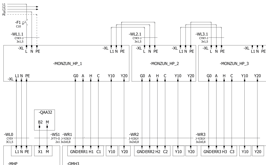
Abb. 4: Anschlusschema der Geräte MONZUN-HP mit der Steuerung OMH3
