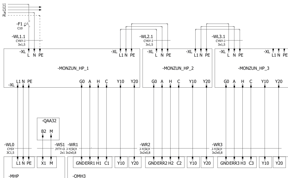
Fig. 4: Schéma de raccordement des groupes MONZUN-HP au boîtier de commande OMH3
