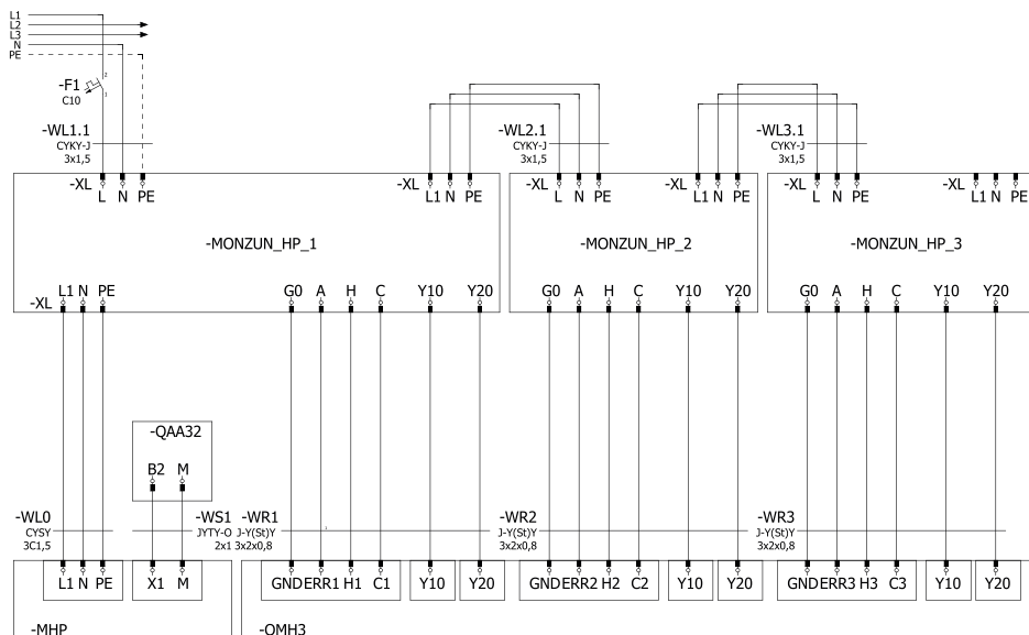
Obr. 4: Schéma propojení agregátů MONZUN-HP s ovládací skříňkou OMH3
