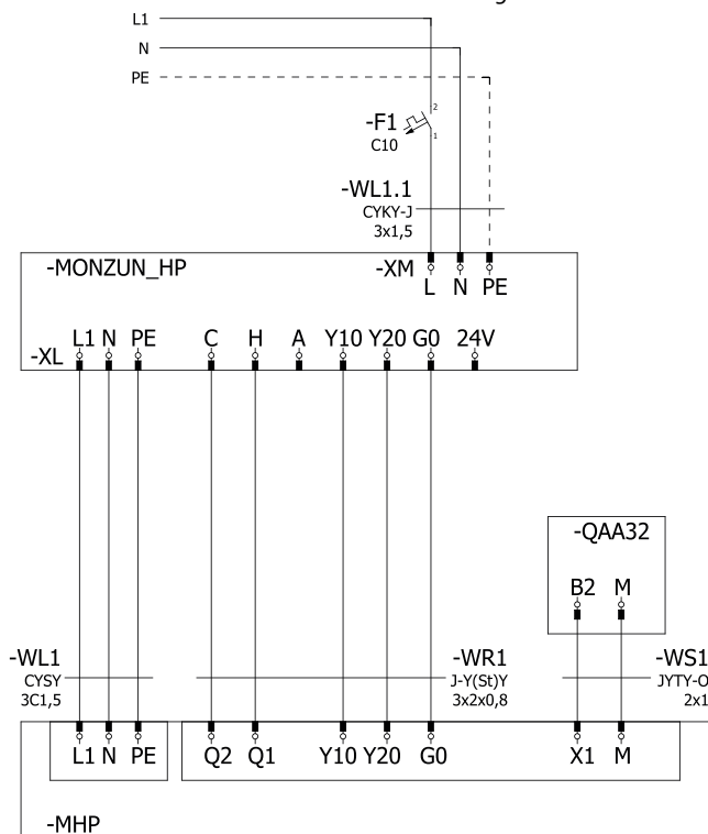
Fig. 2: Schéma de raccordement de l'appareil de chauffage MONZUN au boîtier de commande MHP
