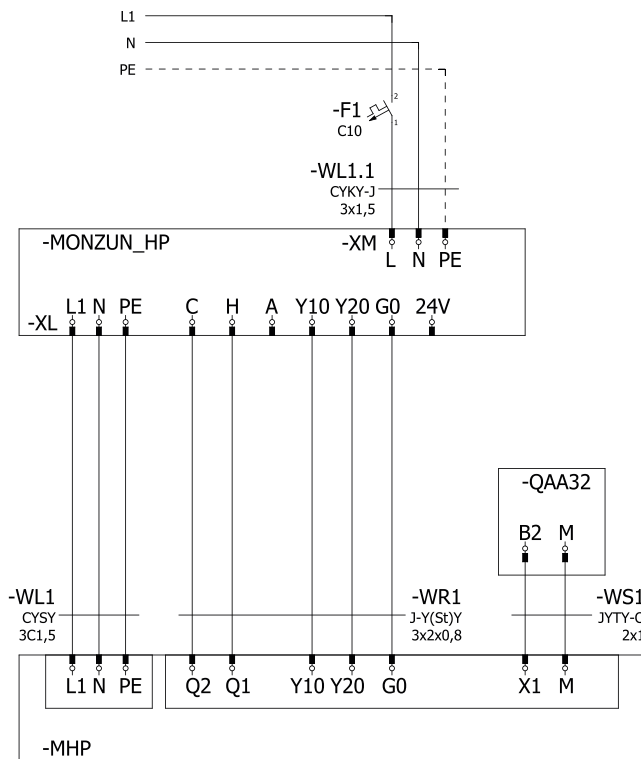
Abb. 2: Schema der Verbindung des Erhitzers MONZUN-HP mit dem Schaltkasten MHP
