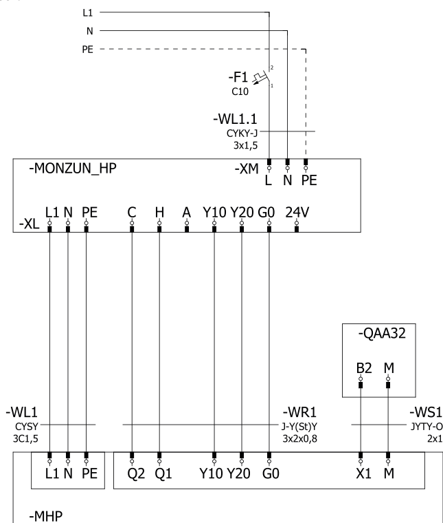
Obr. 2: Schéma propojení ohřívače MONZUN-HP s ovládací skříňkou MHP
