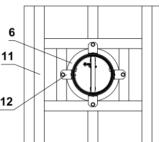
Ansehen B - Raster vom „U“-Profil
