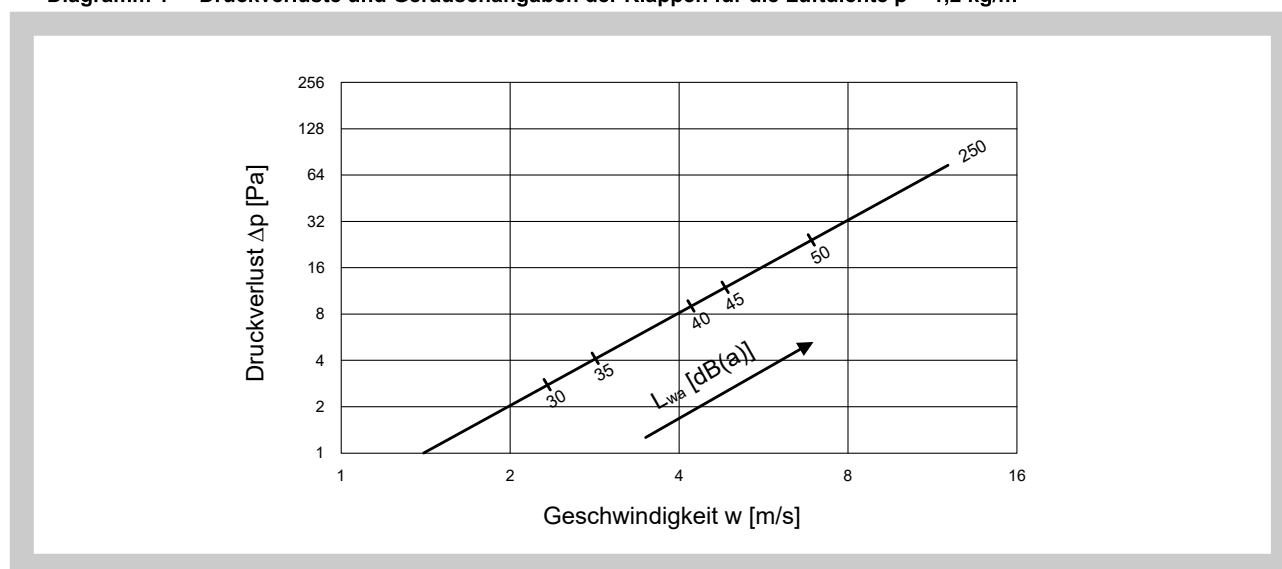
Diagramm 1 Druckverluste und Geräuschangaben der Klappen für die Luftdichte \rho = 1,2 \text{ kg/m}^3
