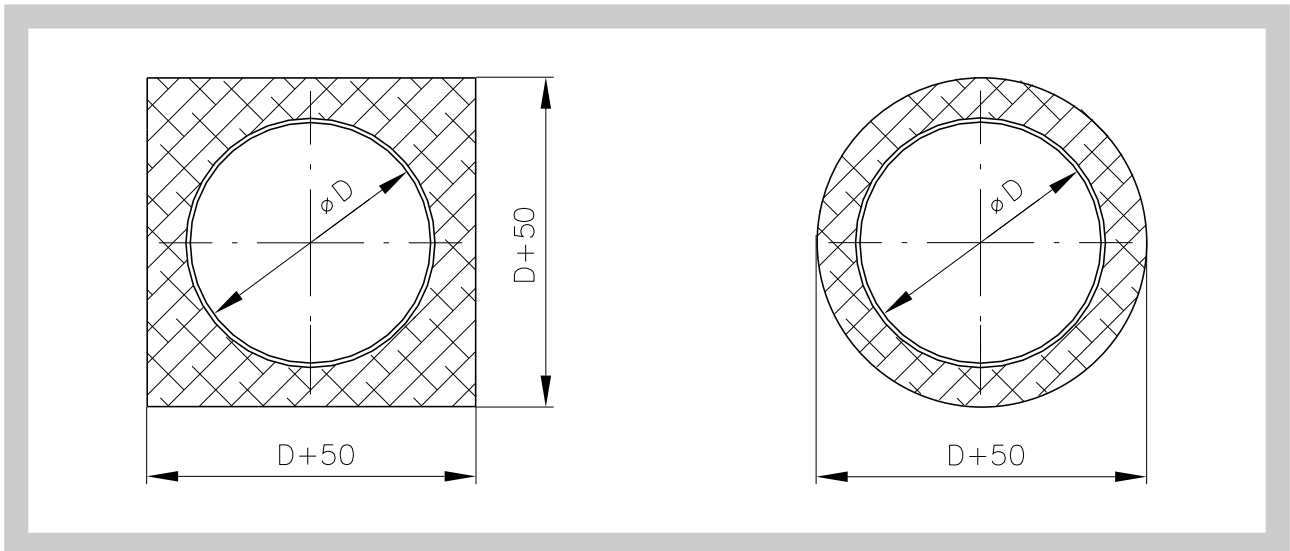
Abb. 8 Bauöffnung
