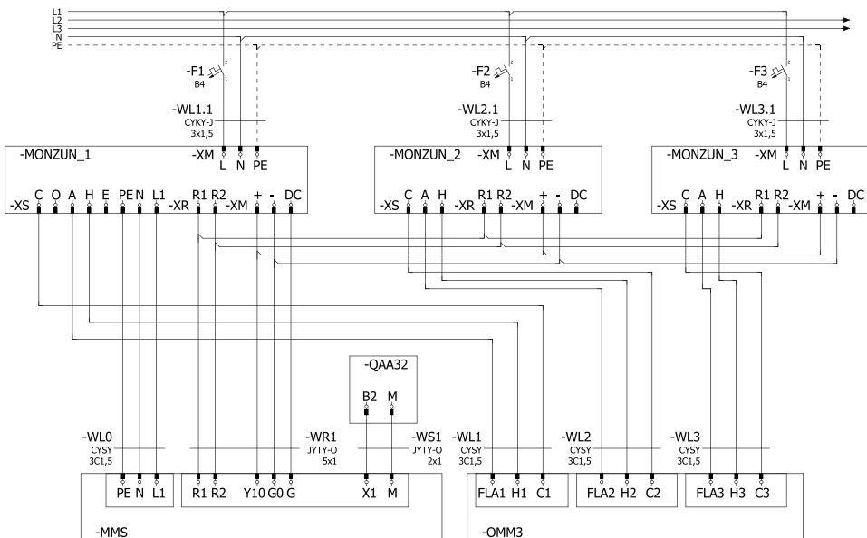
Fig. 4: Schéma de raccordement des groupes MONZUN au boîtier de commande OMM3
