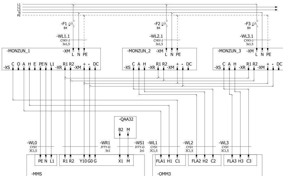
Abb. 4: Anschlusschema der Geräte MONZUN mit der Steuerung OMM3
