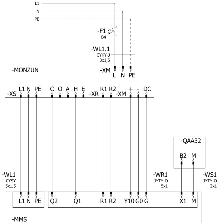
Abb. 2: Schema der Verbindung des Erhitzers MONZUN mit dem Schaltkasten MMS
