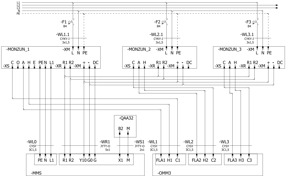
Obr. 4: Schéma propojení agregátů MONZUN s ovládací skříňkou OMM3
