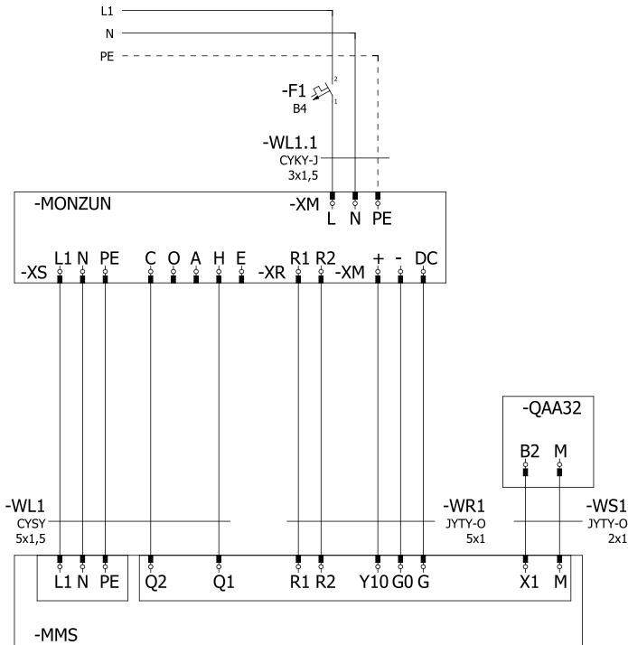
Fig. 2: Schéma de raccordement de l'appareil de chauffage MONZUN au boîtier de commande MMS
