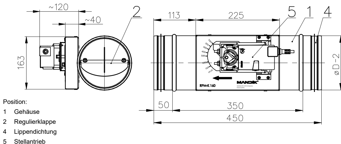
Abb. 4 RPM-K – motorischer Regler
